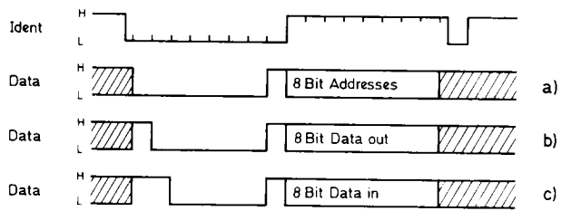
Fig. 8: Signal diagram for the IM bus
