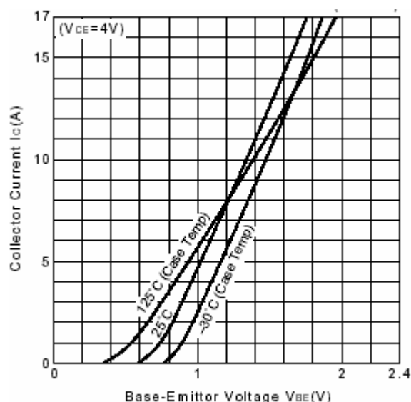
Fig.7 I_C-V_{BE}
