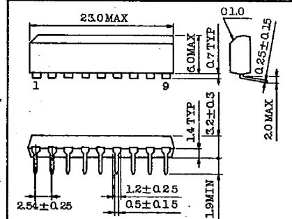
JEDEC — TOSHIBA S9B-P OUTLINE(2)
