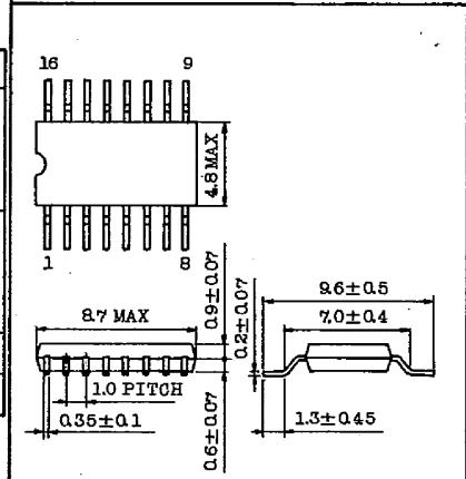
JEDEC — TOSHIBA F16GA1-P OUTLINE(3)
