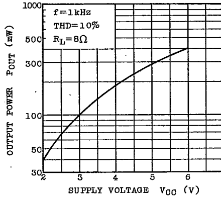
POUT - V_{CC}
