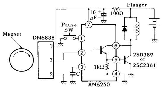
オートリバース回路
