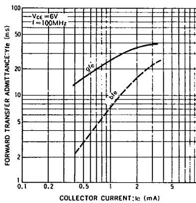
Fig.17 順伝達アドミタンスーコレクタ電流特性
