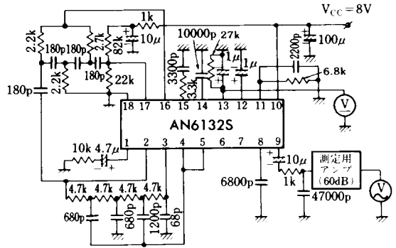
Test Circuit 4 ( V_{no} , V_{AGC} )
