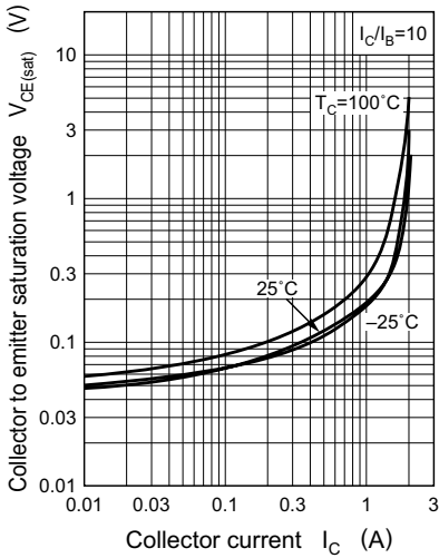
V_{CE(sat)} - I_C
