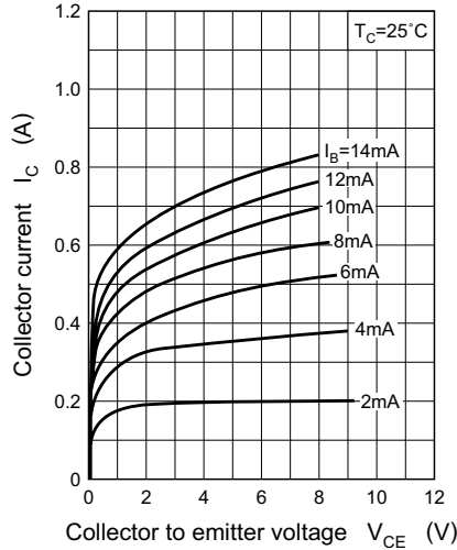
I_C - V_{CE}
