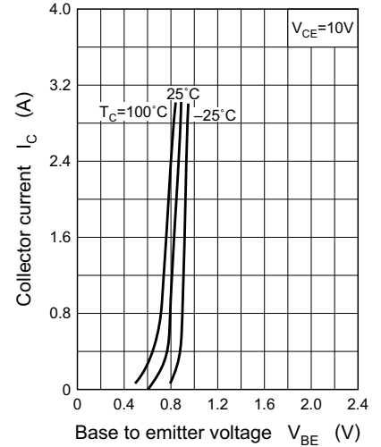
I_C - V_{BE}
