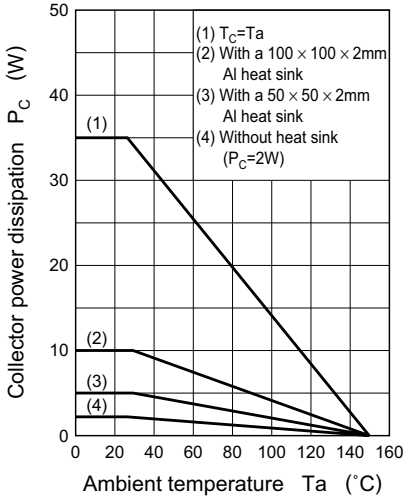
P_C - T_a
