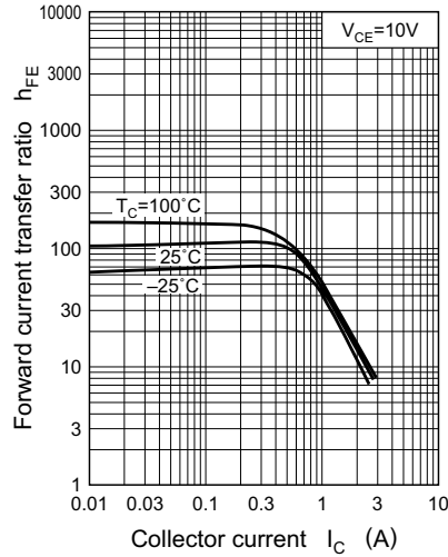
h_{FE} - I_C
