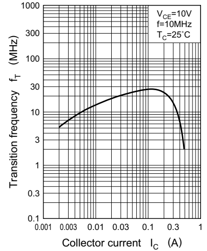
f_T - I_C
